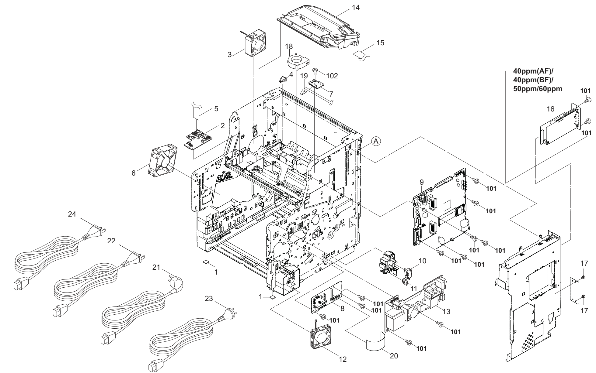
FIG. 2 Frames
