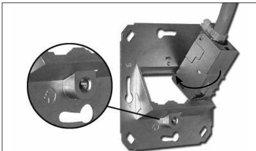
Optional Potentialausgleich Optional potential equalization Compensation de potentiel optionnelle
