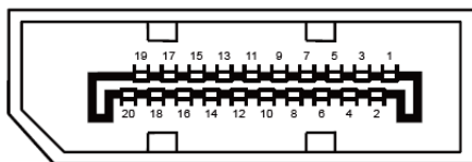
20-nastainen värinäyttösignaalkaapeli
