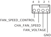
CHA_FAN1/WP
