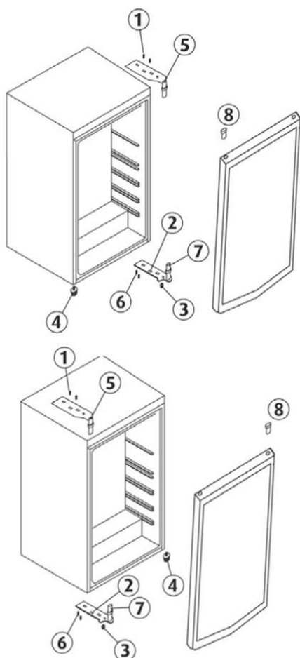
Figur 2 Position av komponenter efter dörrens gångjärn har vänts.
