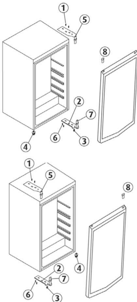
Fig. 2 Placering af komponenter, efter dørhængslet vendes.
