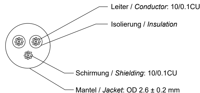
Aderquerschnitt / Wire cross section
