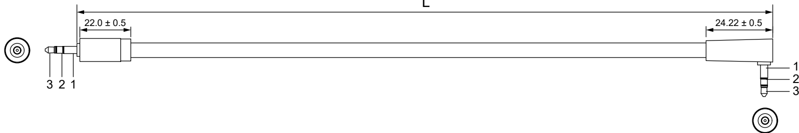
Anschlussdiagramm / Wiring diagram
