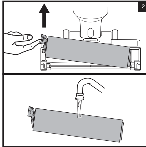
2. Fjern børsterullen ved å trekke opp på trekkefanen på venstre side av munnstykket.
