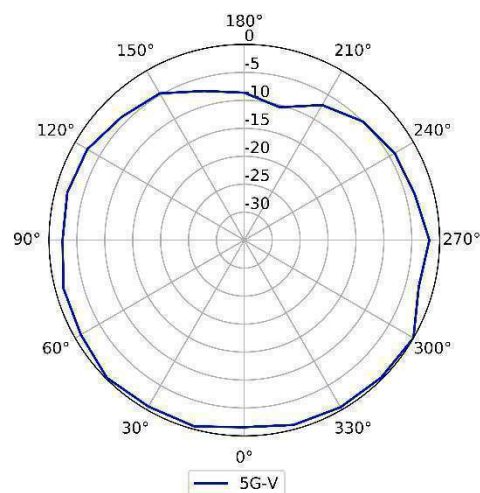
5GHz (Vertical)
