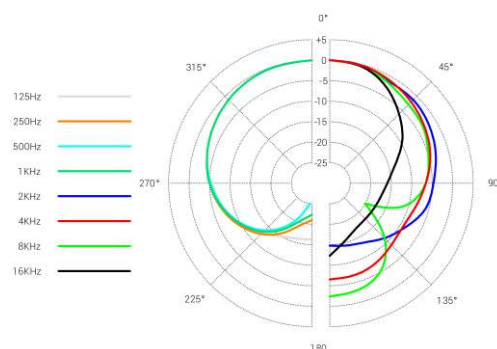
Polaridiagramm
