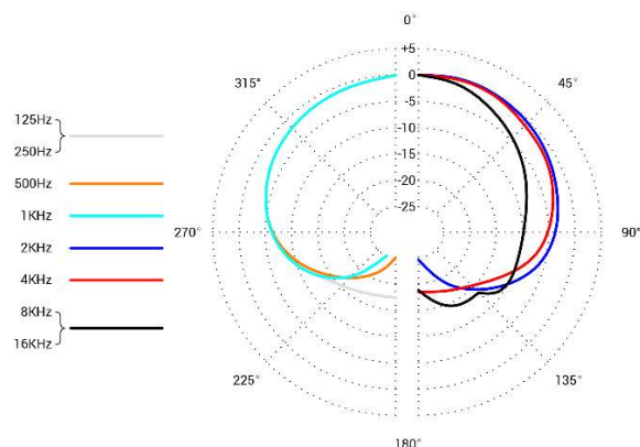
指向性
