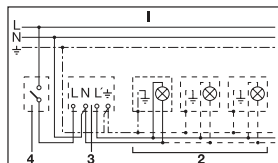
1. Lámpara sin conductor neutro
