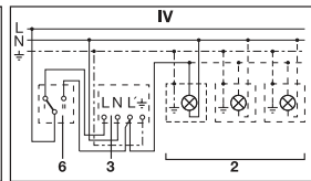
2. Armatur med nolledaren ansluten via sensorn.
