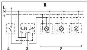
2. Candeiro com neutro
