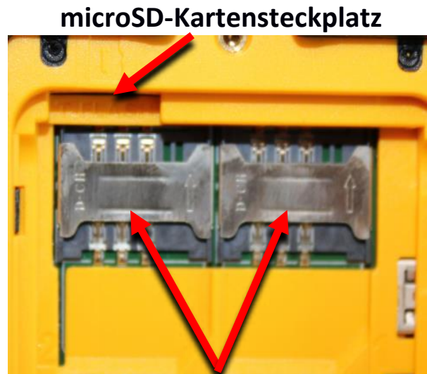
SIM-Kartensteckplatz
