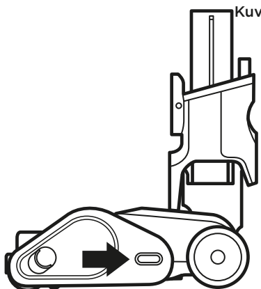
EDGEDETECT-REUNANTUNNISTUSANTURI
