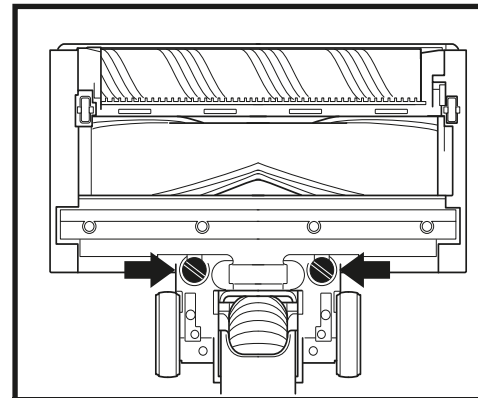
VEDENPURISTUSTELAN IRROTTAMINEN
