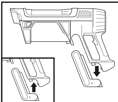
REMOÇÃO DA BATERIA
