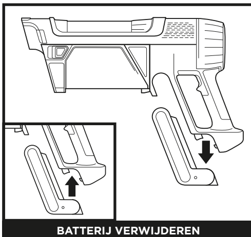
BATTERIJ VERWIJDEREN
