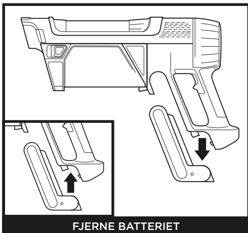
FJERNE BATTERIET
