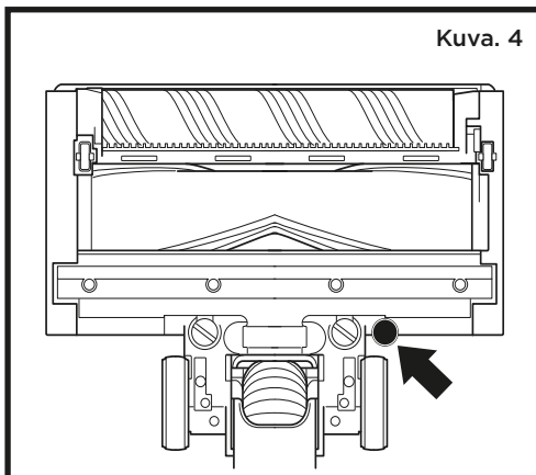
FLOORDETECT- LATTIANTUNNISTUSANTURI
