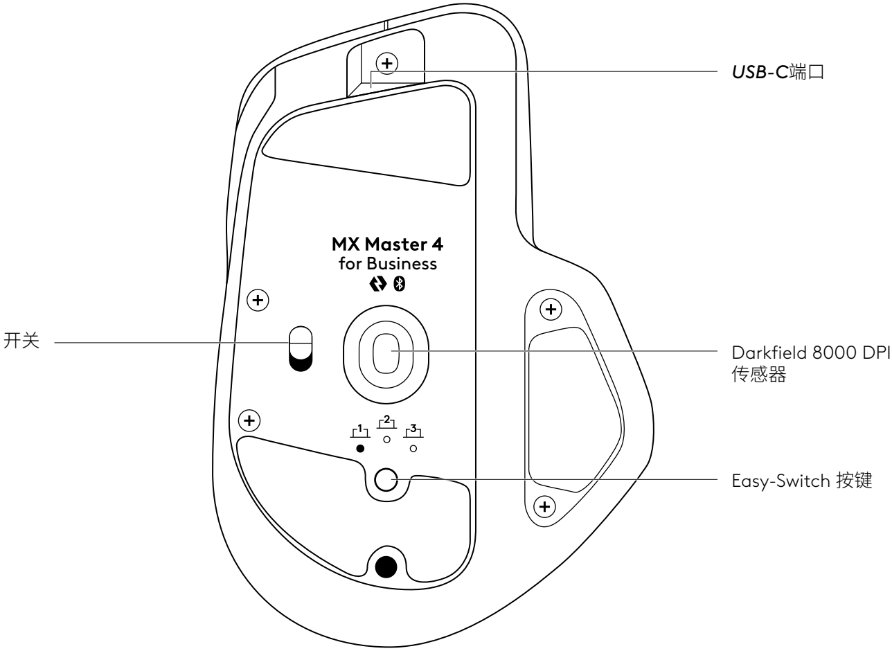
后视图
