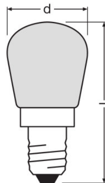
SPC.T FR 15 W 230 V E14, SPC.T FR 25 W 230 V E14
