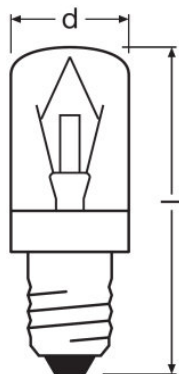
SPC.T CL 15 W 230 V E14
