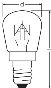
SPC.T CL 15 W 230 V E14, SPC.T CL 25 W 230 V E14
