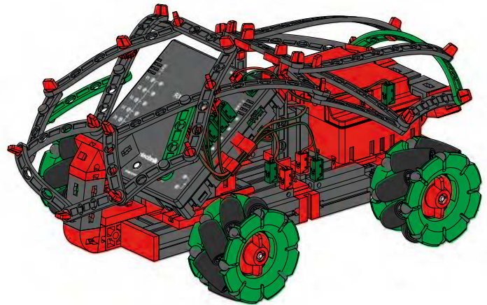
Omnwheels Basismodell / Omniwheels Base Model / Omniwheels Modèle de base / Omniwheels Base Model / Omniwheels Modelo básico / Omniwheels Modelo básico / Omniwheels Modello base / Omniwheels Базовая модель / 全能轮基本型号 ..... 62
