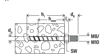
Typ M8/M10
