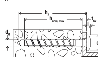
Typ LP
