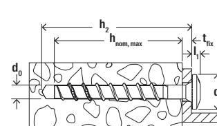
Typ P
