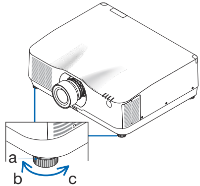
a: Tilt foot / b: Up / c: Down
