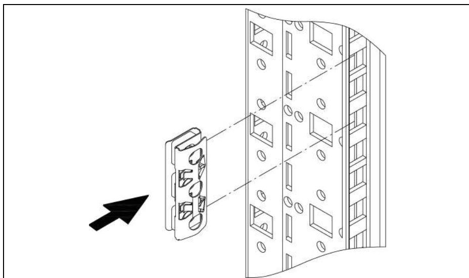
Abb./Fig./Fig. 2: Montage Käfigmutter / Fitting the cage nuts / Montage de l'écrou cage
