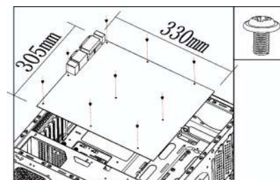
Einbau Mainboard auf dem Träger
