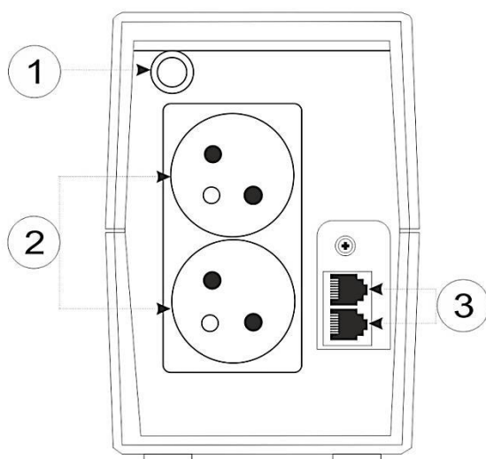
Rysunek 2: Elementy panelu tylnego EASYLINE 650 / 850 AVR USB .
