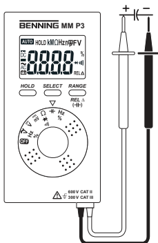
Bild 7: Kapazitätsmessung
