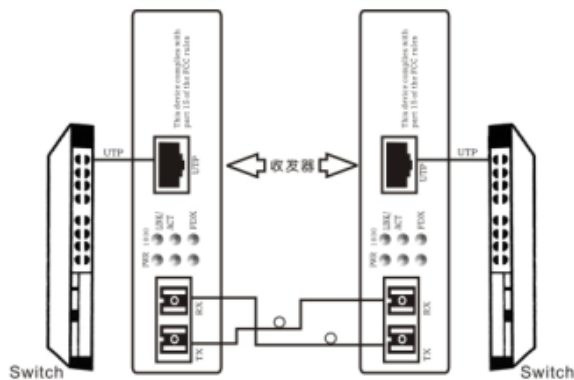
Abbildung 5.1 MC Anschlussdiagramm
