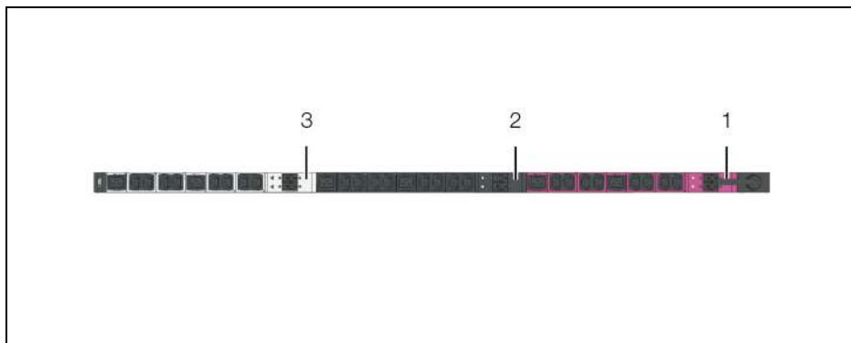
Abb./Fig./Fig. 12: Farbkenngng der einzelnen Phasen und Steckplätze / Colour coding of individual phases and slots / Codage couleur des différentes phases et fentes
