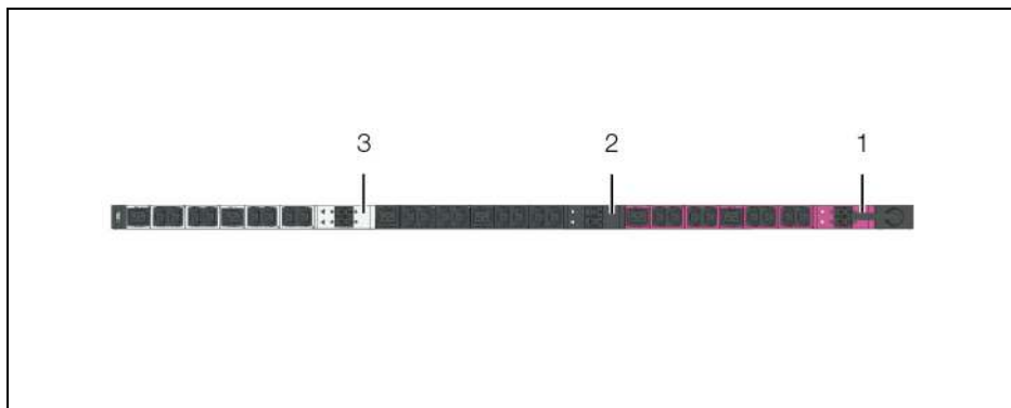
Abb./Fig./Fig. 12: Farbkenngung der einzelnen Phasen und Steckplätze / Colour coding of individual phases and slots / Codage couleur des différentes phases et fentes
