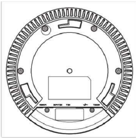
GWN7610/GWN7600 Ports
