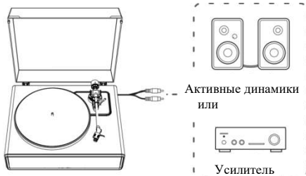
Проводное подключение RCA
