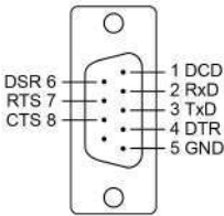
RS-232
