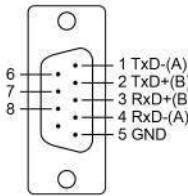
RS-422/RS-485-4w
