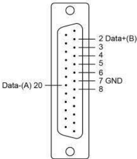
RS-485-2w
