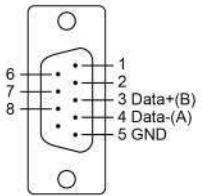
RS-485-2w
