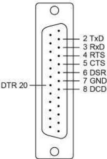
RS-232
