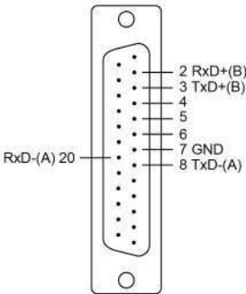
RS-422/RS-485-4w
