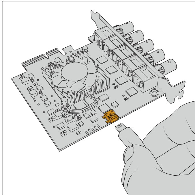
DeckLink 카드를 컴퓨터의 PCIe 슬롯에서 제거한 다음 카드 뒷면 또는 측면의 USB-C 또는 미니 B USB 포트를 사용해 컴퓨터와 연결하세요.
