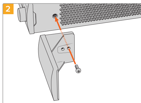
Выровняйте заглушку и закрепите ее с помощью прилагаемого 9-мм винта M3
