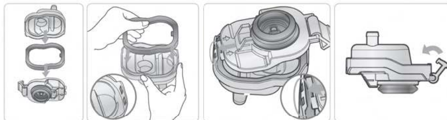
스팀캡 분해도
